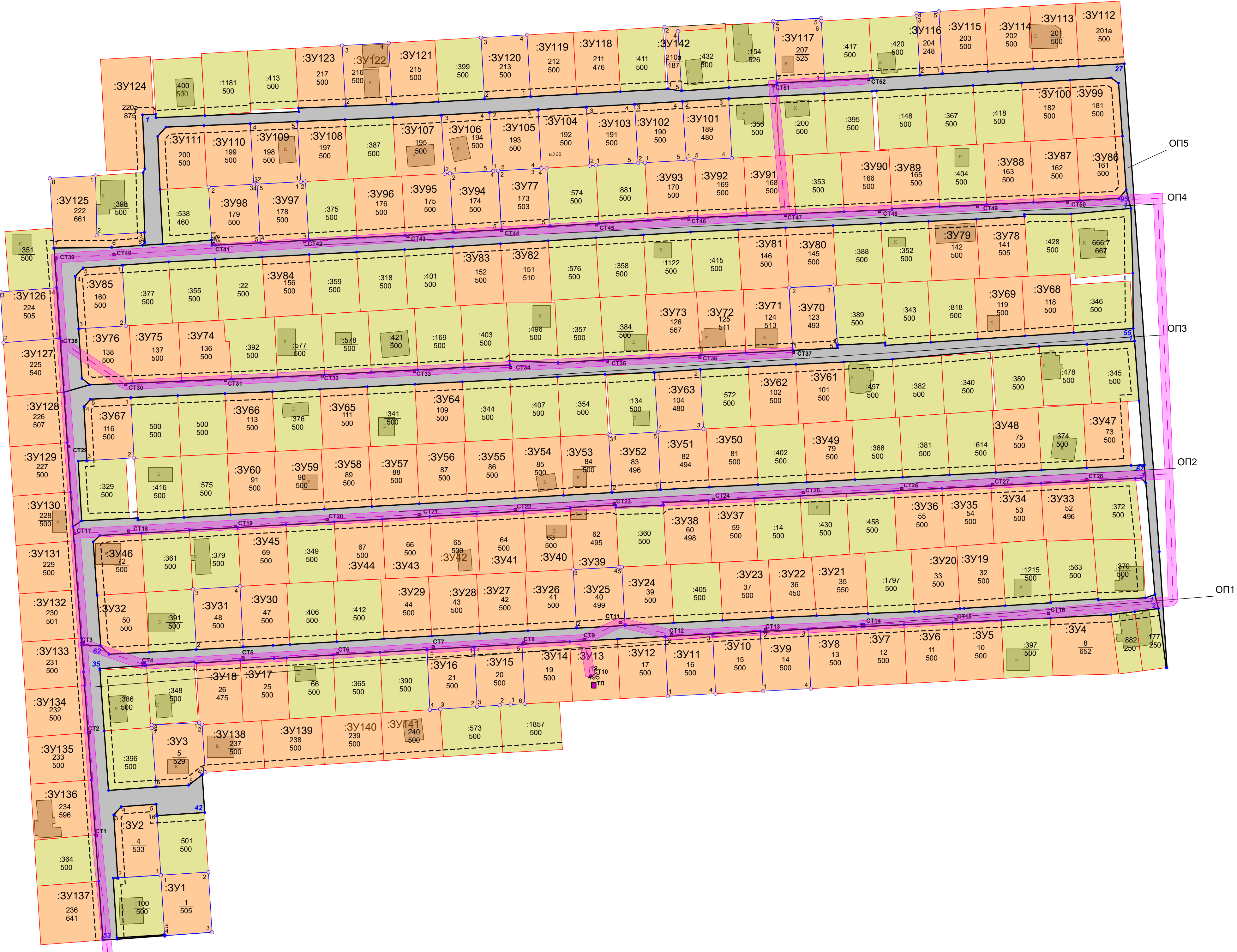
План межевания территории Т СН "Кипарис" М 1:1000
